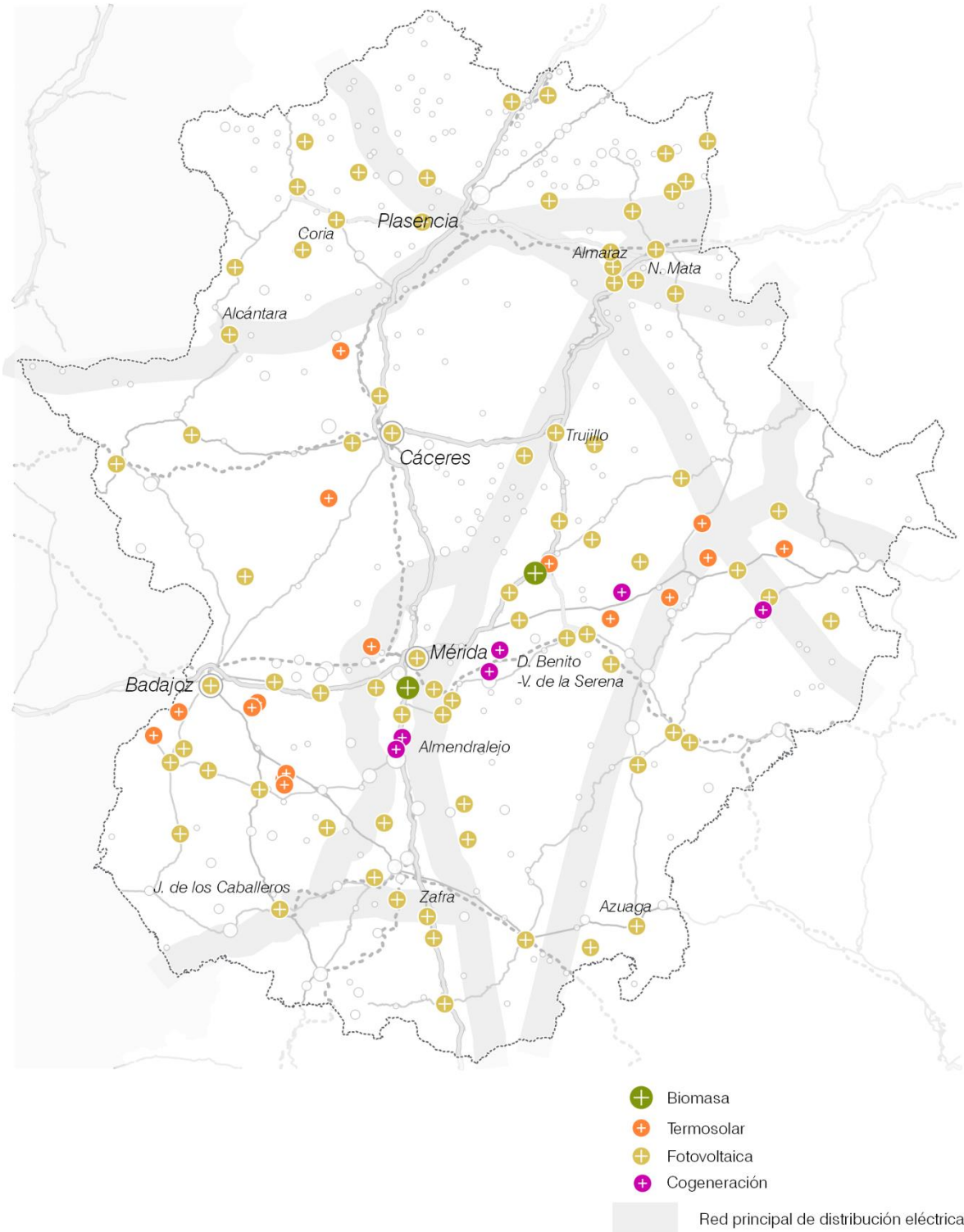
Mapa 65. Fuentes de energía renovables. Consejería de Agricultura, Desarrollo Rural, Medio Ambiente y Energía.
