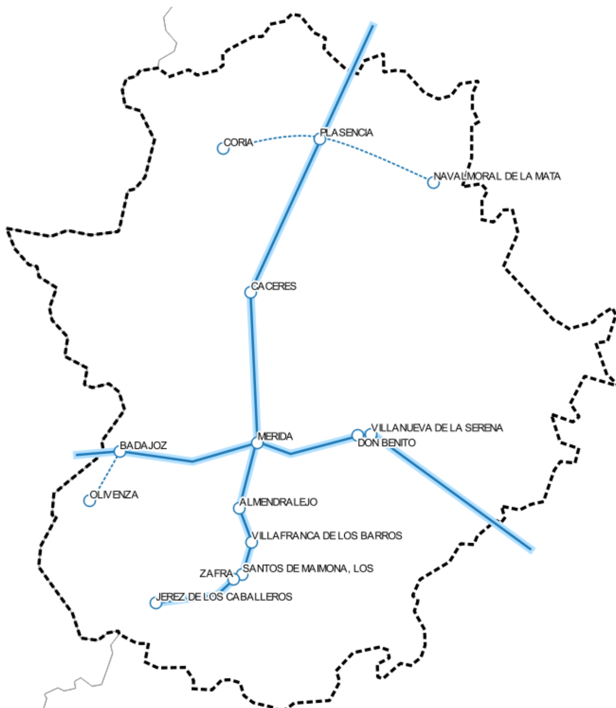
Mapa 41. Esquema de la red gasista
