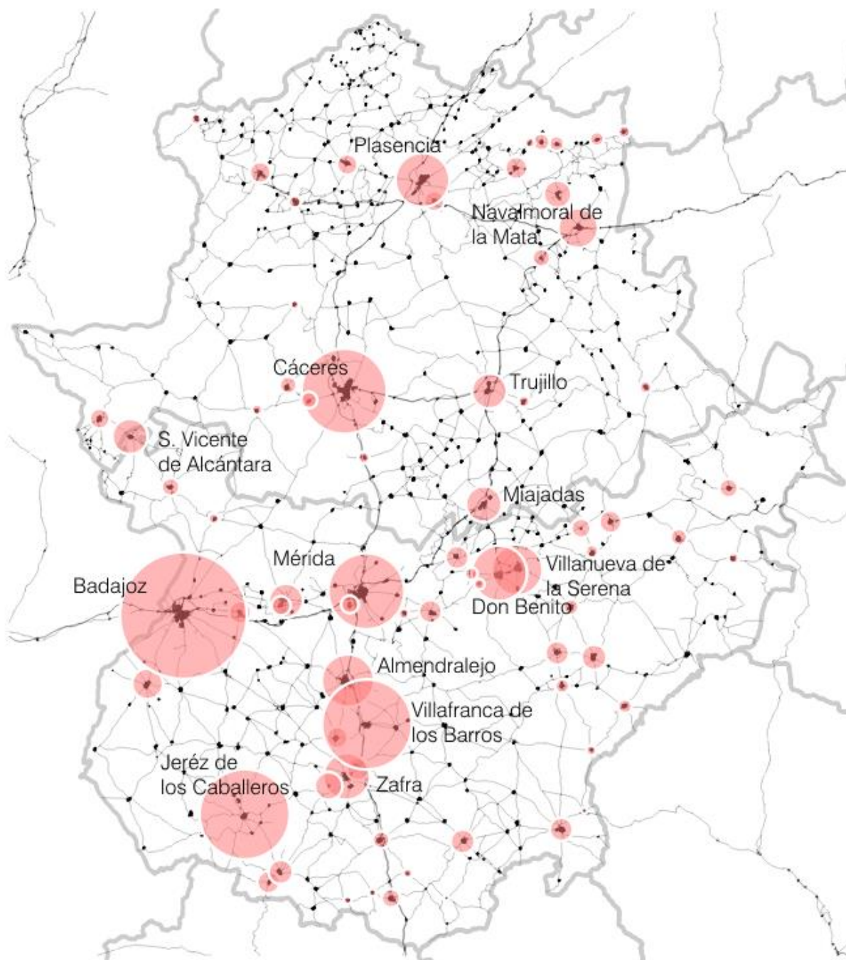
Mapa 66. Puntos de mayor consumo eléctrico en la región (tamaño del círculo proporcional al consumo anual). Consejería de Agricultura, Desarrollo Rural, Medio Ambiente y Energía.
